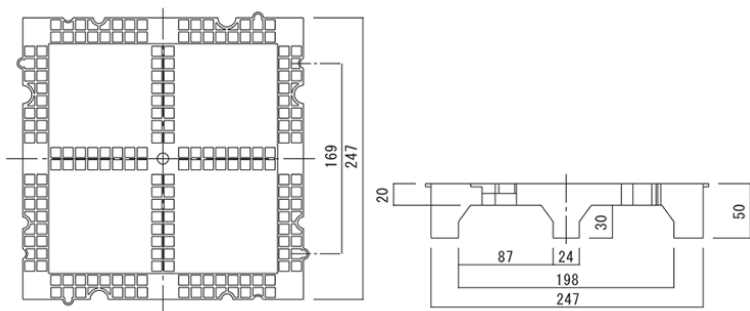
寸法図
